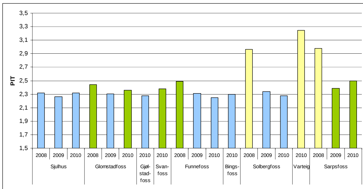
Figur 9. Gammel eutrofieringsindeks PIT (Periphyton Index of Trophic status) beregnet for 8 stasjoner fra Sjulhus til Sarpsfoss langs Glomma og Svanfoss i Vormå, der PIT-verdiene angir økologisk tilstand. Blå = svært god, grønn = god, gul = moderat tilstand.
