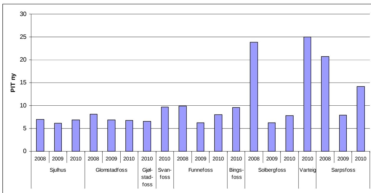
Figur 10. Ny PIT (Periphyton Index of Trophic status) beregnet for 9 stasjoner fra Sjulhus til Sarpsfoss langs Glomma og Svanfoss i Vormå, der PIT-verdiene i relativ forstand angir økologisk tilstand. Lave verdier indikerer god økologisk tilstand, mens høyere verdier indikerer dårligere tilstand.
