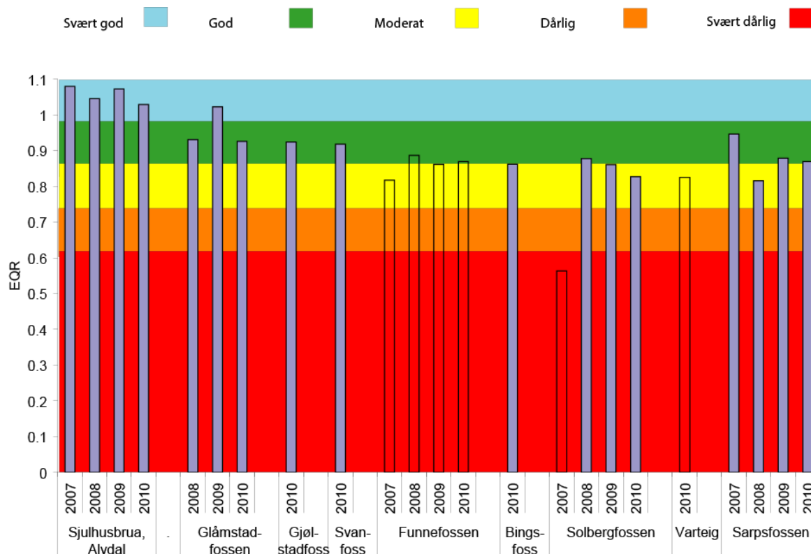
Figur 13. Økologisk tilstand basert på bunndyr ved stasjoner i Gomma 2007 – 2010 og Svanfoss i Vormå i 2010. Åpne søyler angir habitattyper som ikke er med i klassifikasjonssystemet
