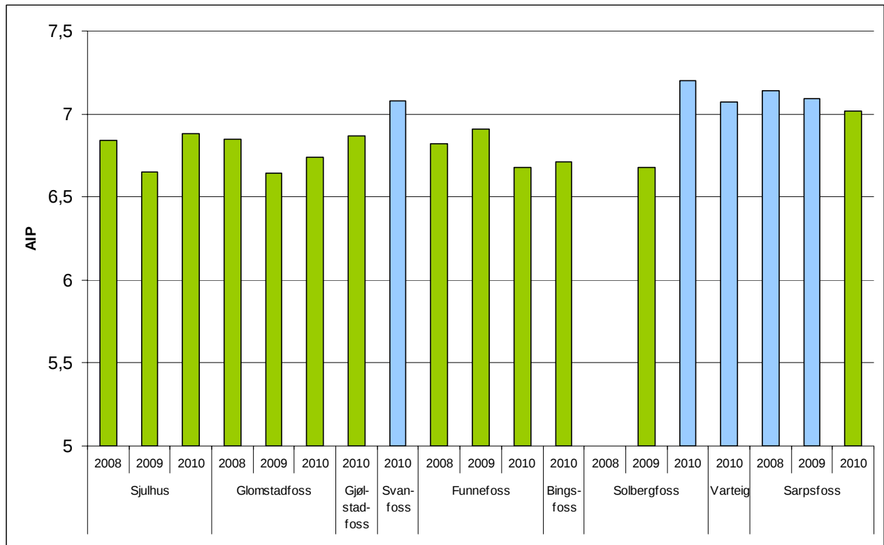
Figur 11. Forsuringsindeks AIP (Acidification Index for Periphyton) beregnet for 9 stasjoner fra Sjulhus til Sarpsfoss langs Glomma og Svanfoss i Vorma, der AIP-verdiene angir økologisk tilstand. Blå = svært god og grønn = god tilstand.
